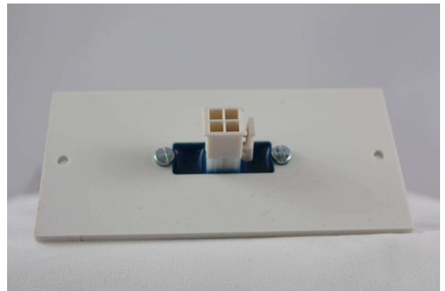
Bezeichnung: MAS-Adapter MiniFit 4pol Art.Nr. MAS-MiniFit-4
